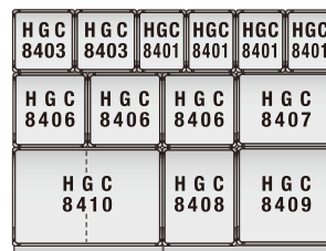
UNIT 9 幅2,730mm／高さ2,090mm
