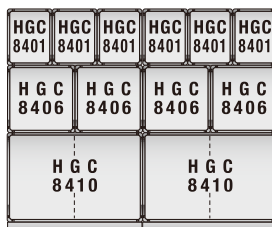
UNIT 8 幅2,520mm／高さ2,090mm
