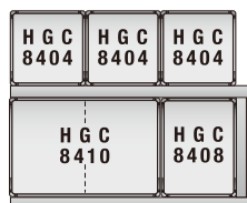
UNIT 22 幅1,990mm／高さ1,600mm
