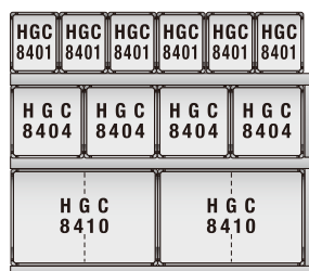
UNIT 31 幅2,620mm／高さ2,180mm
